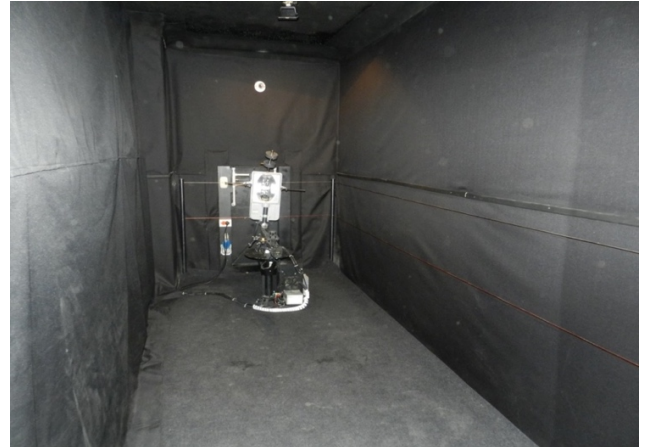
Figura 14. Laboratorio Aplicado de Iluminación
